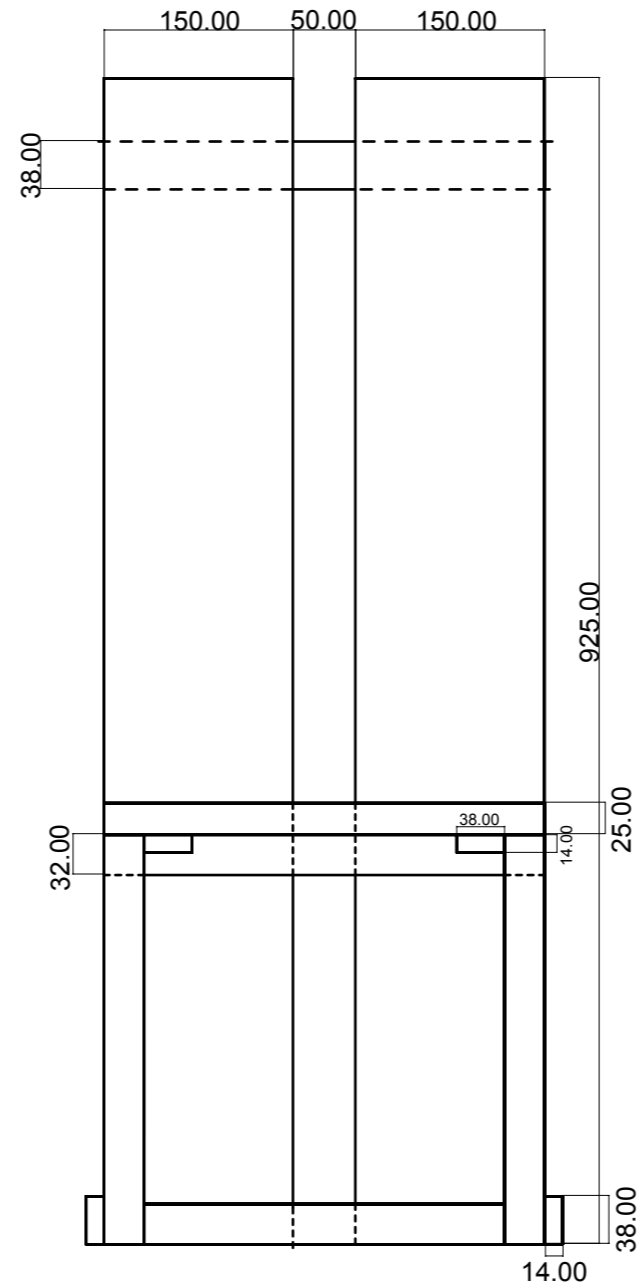
Vue de face / Front view Échelle / Scale 1/6
