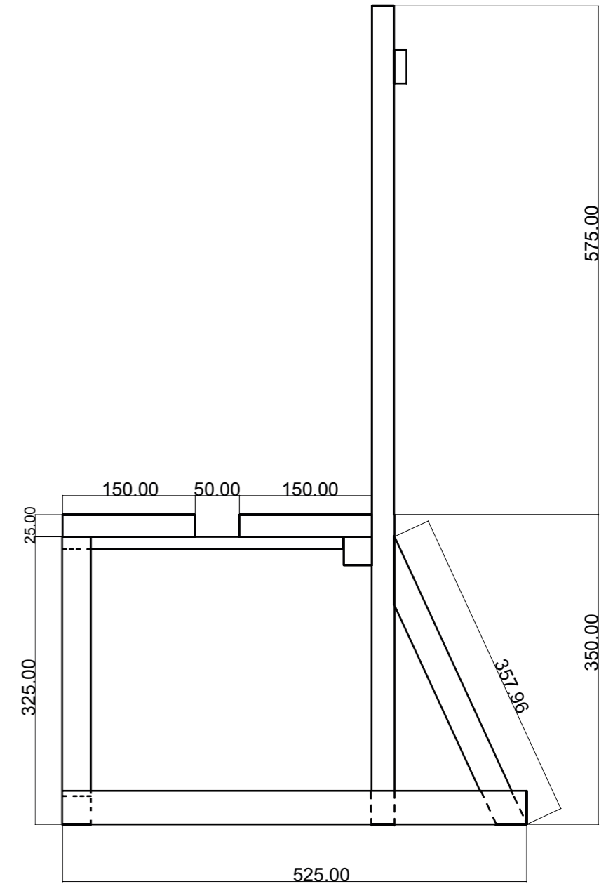
Vue de droite / right view Échelle / Scale 1/6
